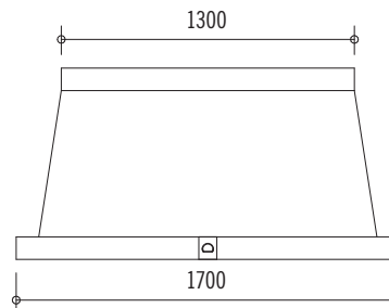
HOTTE CHÂTEAU 150 : H1770 L 1700 x H 850 x P 650 (mm)
